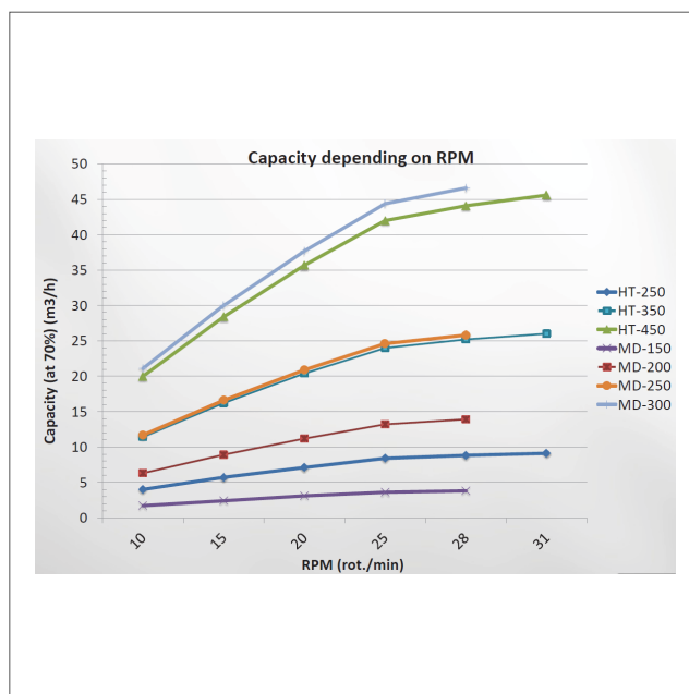
Kapacitetsdiagram för rotorslussar HT/HT-S/MD
