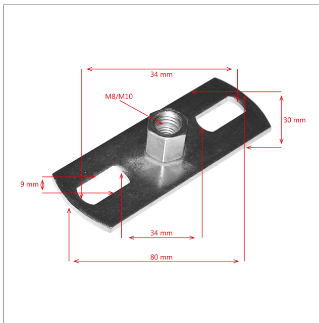
GRFL - Fästplatta - måttskiss
